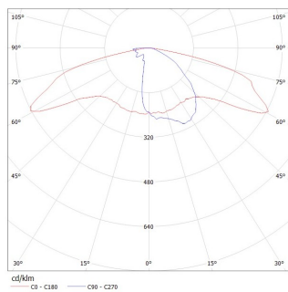
Кривая распределения силы света Светильника «Сириус.м»
