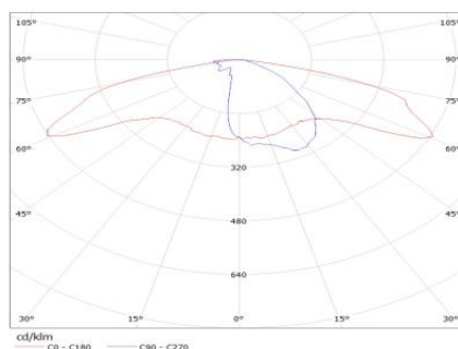
Фото и кривая силы света светильника РКУ 11-250 LED-1
